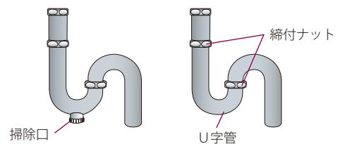
掃除口のある場合
