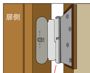
●上下調整ネジ
