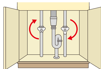
洗面台やキッチンの下にある止水栓を閉めると水の供給が止まります。
