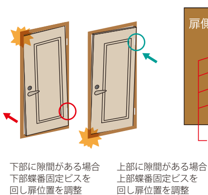
●蝶番固定ビス
